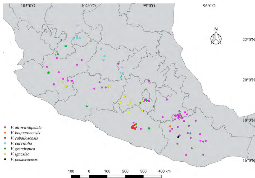
Figura 3. Mapa de distribución de Viridantha atroviridipetala , V. boqueronensis , V. caballoensis , V. curvifolia , V. grandispica , V. ignesia y V. penascoensis .
