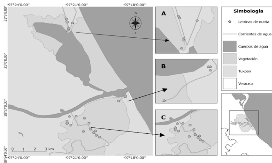
Figura 1. Distribución de letrinillas de la nutria neotropical en los sitios de muestreo en la zona costera de Tuxpan, Veracruz. (A) Laguna de Tampamachoco; (B) estero Jácome y (C) estero Tumilco.
